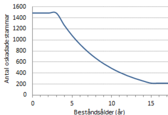
Figur 5. Prognos av antalet tallstammar utan viltbetesskador i ett genomsnittligt bestånd. Beräkningarna utgår från skattat antal stammar per ha (data 2009-2014) och skattad skaderisk (data 2014).
